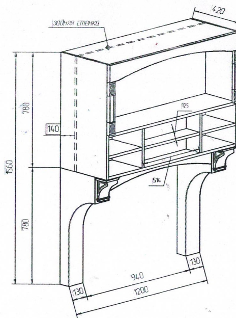
ПОРТАЛ №3 (труба вытяжки \phi 150\text{мм.} ) более расширенный вариант вытяжек!!!
